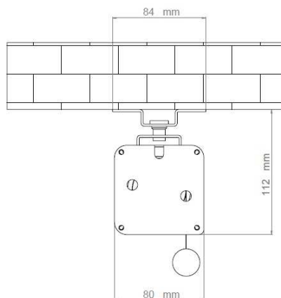
Fissaggio a soffitto
