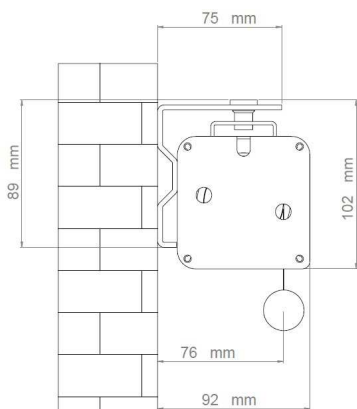
Fissaggio a parete con caduta tela anteriore
