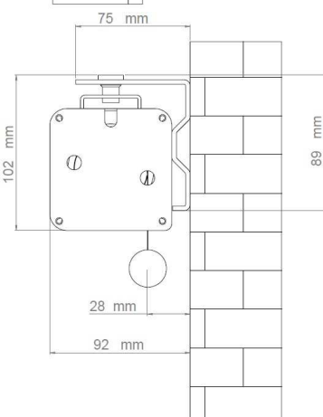
Fissaggio a parete con caduta tela posteriore
